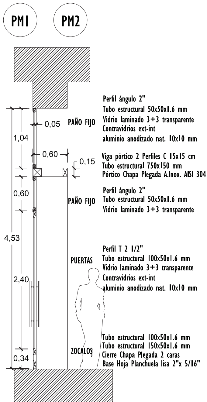
ESQUEMA SECCION CONSTRUCTIVA PUERTAS CIERRE PMI - PM2
